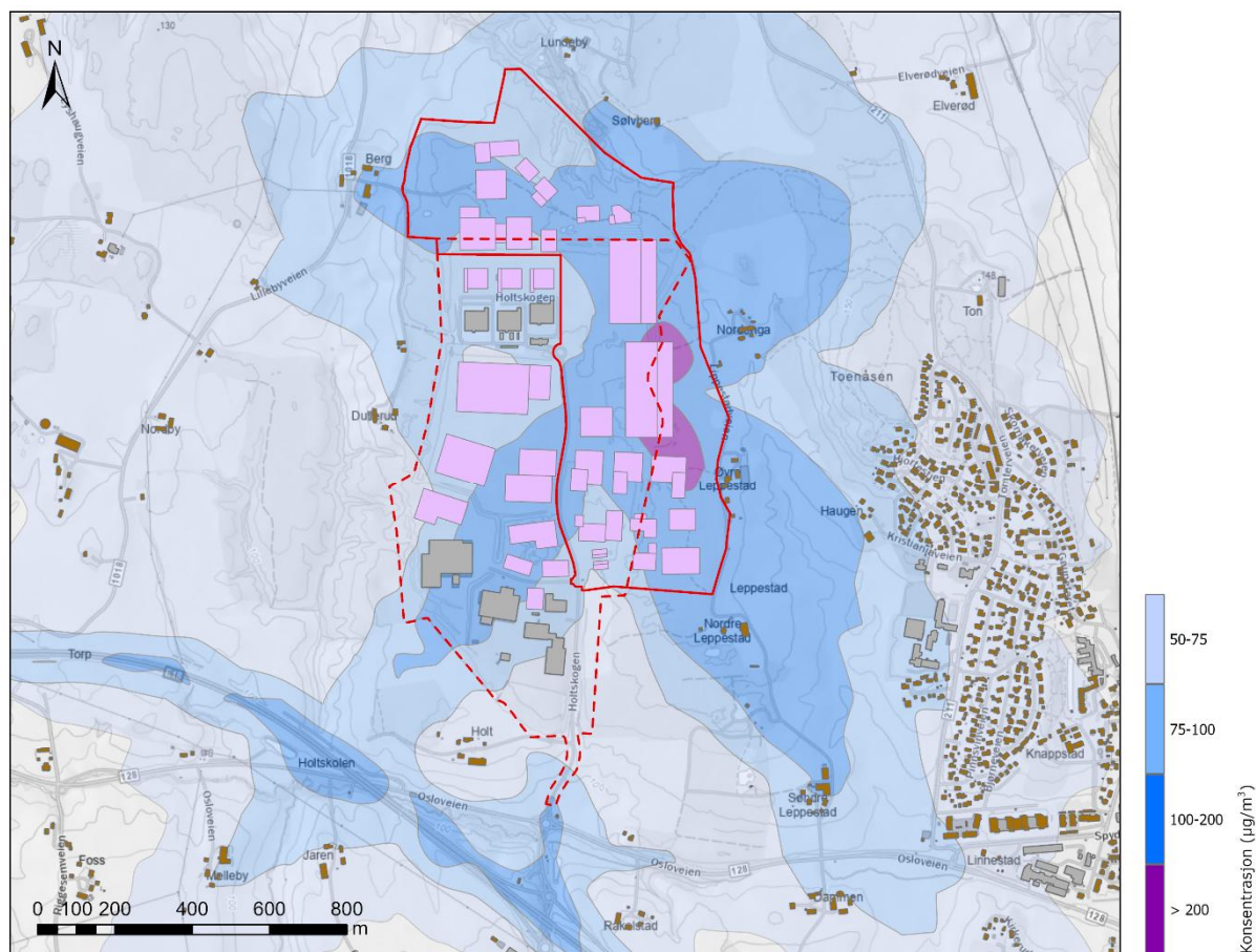
Figur 12. Beregnede konsentrasjoner av nitrogendioksid (NO 2 ) som 12. høyeste timemiddel, ved nødkjøring av back up-generatorene tilhørende datasentrene for planforslaget for Holtskogen næringsområde. Grenseverdien for NO 2 som timemiddel er på 200 µg/m 3 med tillatt 3 overskridelser pr. år i revidert EUs luftkvalitetsdirektiv.
