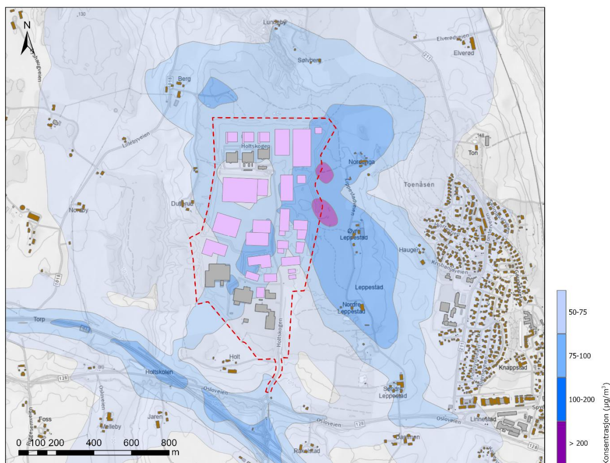
Figur 10. Beregnede konsentrasjoner av nitrogendioksid (NO 2 ) som 12. høyeste timemiddel, ved nødkjøring av back up-generatorene tilhørende datasentrene for nullalternativet for Holt skogen næringsområde, vist for et større område (øverst), og zoomet inn ved næringsområdet (nederst). Grenseverdien for NO 2 som timemiddel er på 200 µg/m 3 med tillatt 3 overskridelser pr. år i revidert EUs luftkvalitetsdirektiv.
