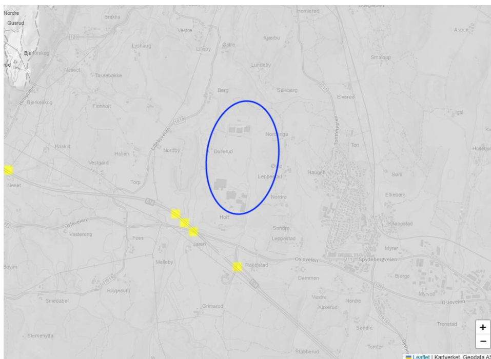
Figur 8. Luftsonerkart som viser utbredelsen av Retningslinje T-1520 rød og gul sone ved Holtskogen, beregnet med meteorologi for årene 2019-23, tatt fra Luftkvalitet i Norge (Miljødirektoratet, 2025a). Omtrentlig plassering til planområdet er markert med blå sirkel.
