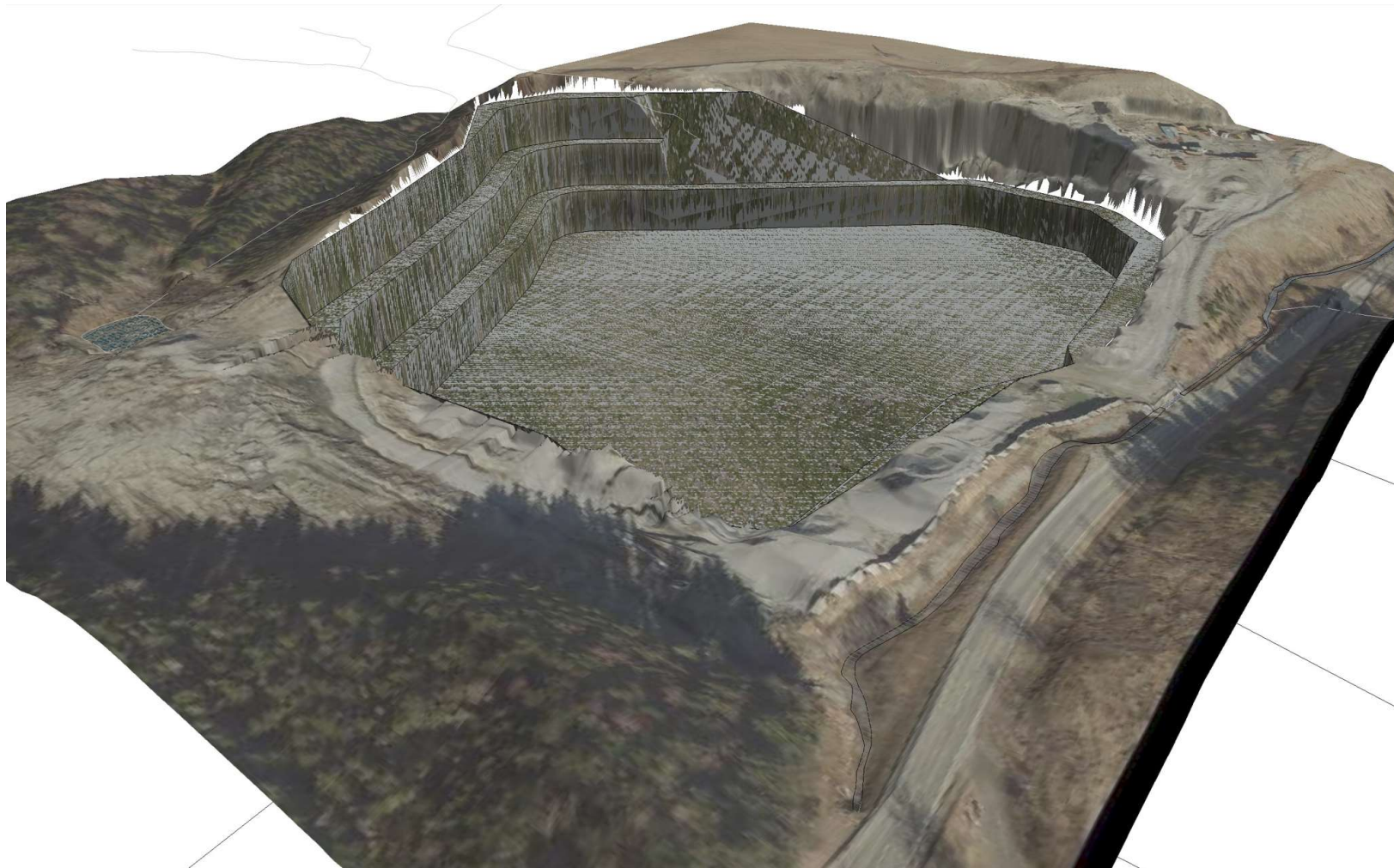
Fig 2a: Avslutning av steinuttak ved kote +63 og angivelse av pallehøyder 14 m og bredde 8 m, sett fra sør.
