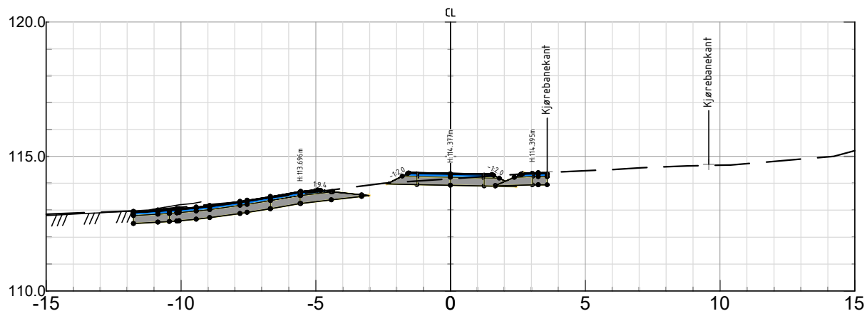
GS1 Pel nr 160 - Skala 1:200
