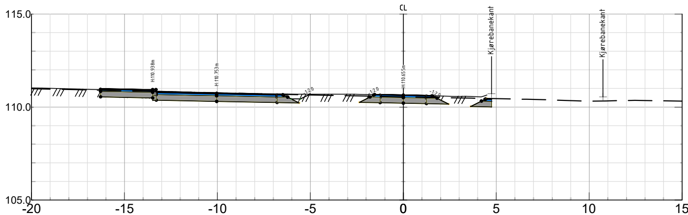
GS1 Pel nr 40 - Skala 1:200
