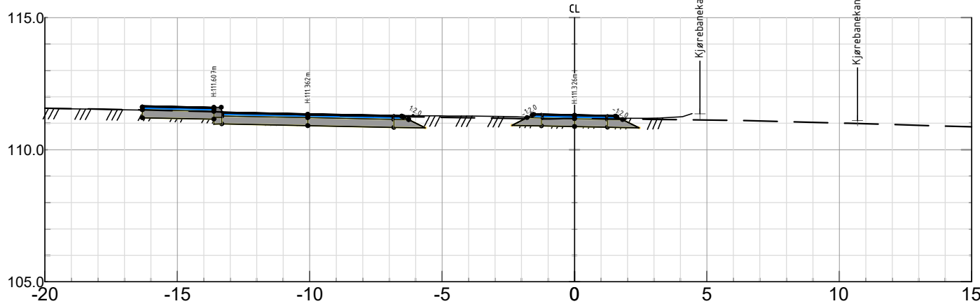
GS1 Pel nr 70 - Skala 1:200
