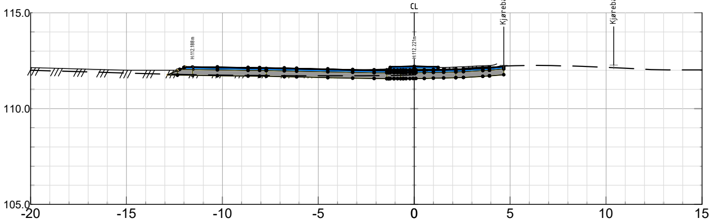
GS1 Pel nr 110 - Skala 1:200
