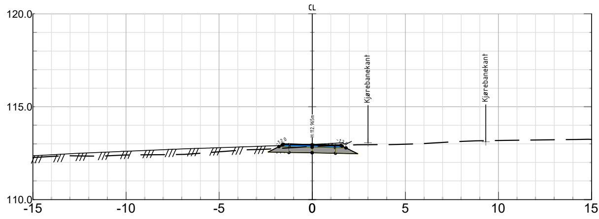
GS1 Pel nr 130 - Skala 1:200
