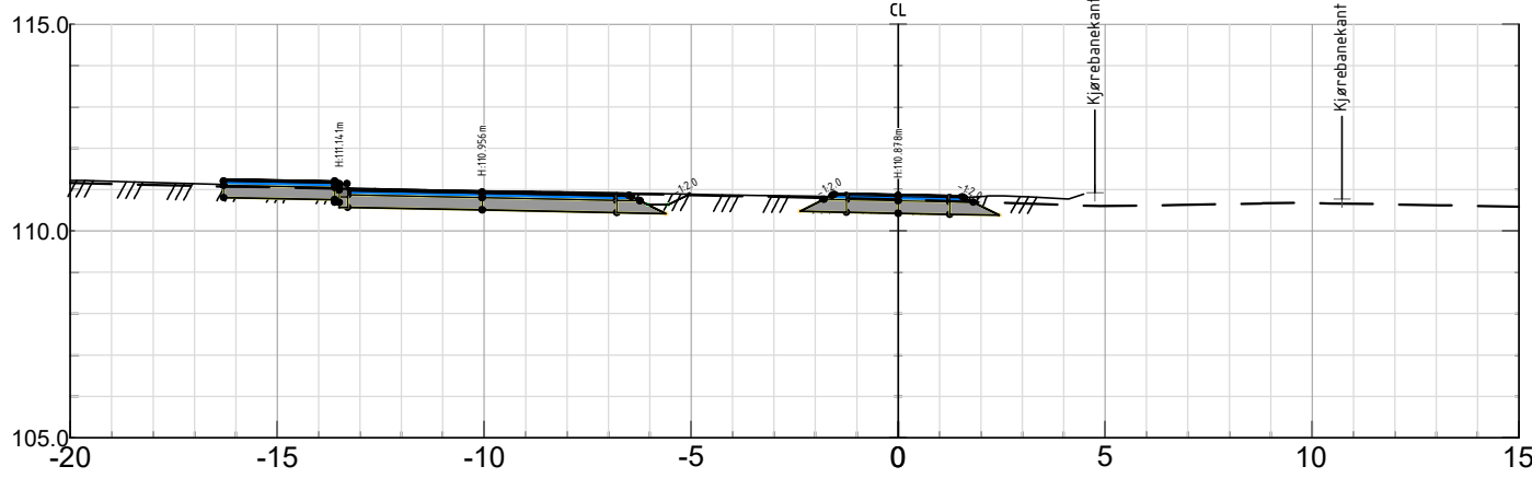
GS1 Pel nr 50 - Skala 1:200
