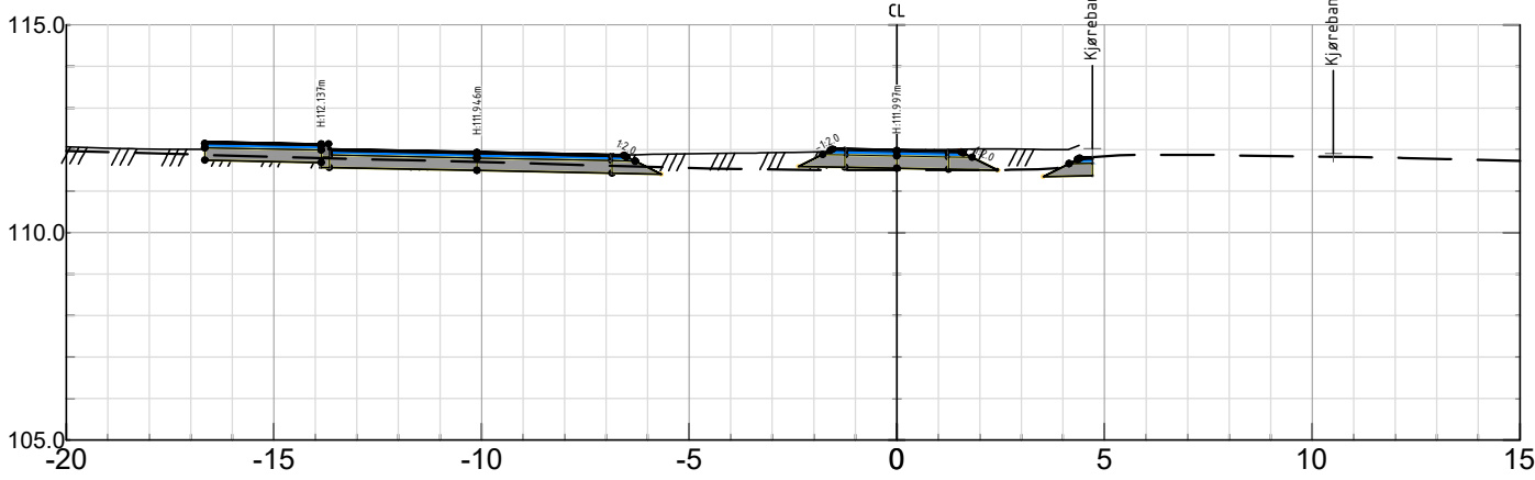
GS1 Pel nr 100 - Skala 1:200
