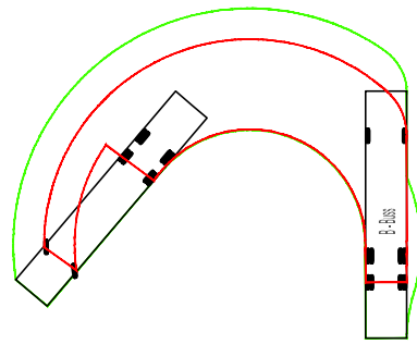
Sporingskurve Buss (15m)
