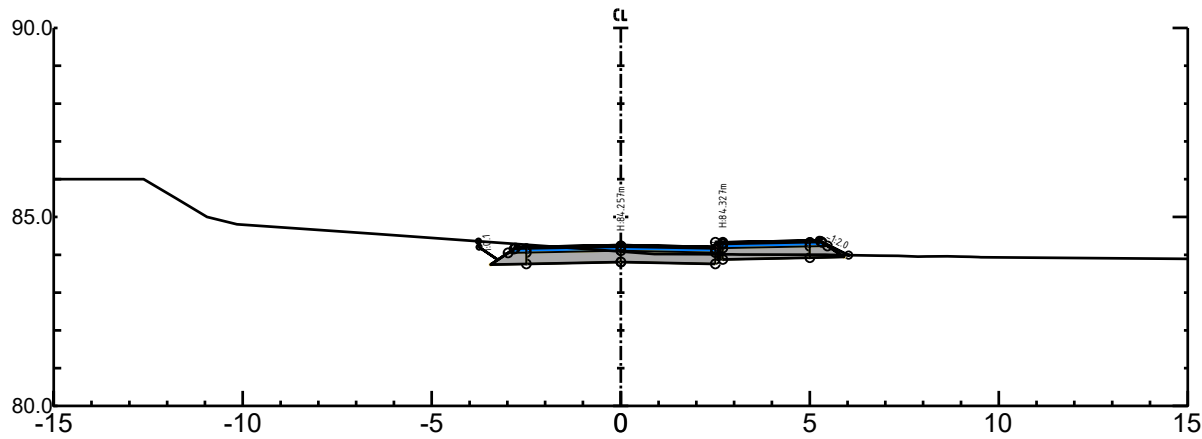
o_V1 Pel nr 130 - Skala 1:500
