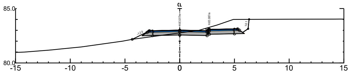
o_V1 Pel nr 270 - Skala 1:500
