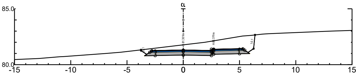
o_V1 Pel nr 310 - Skala 1:500
