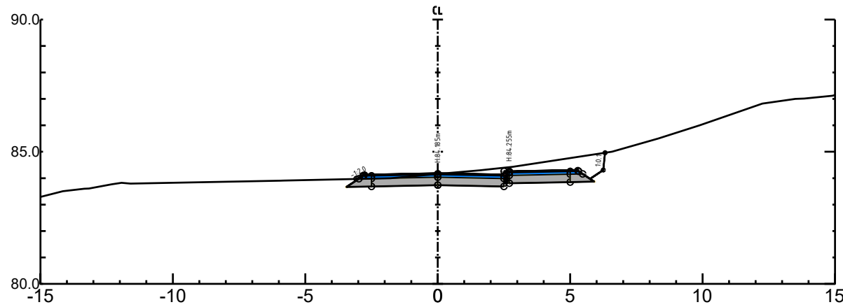
o_V1 Pel nr 210 - Skala 1:500
