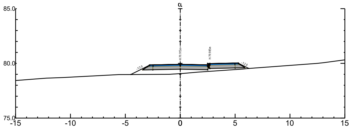
o_V1 Pel nr 380 - Skala 1:500
