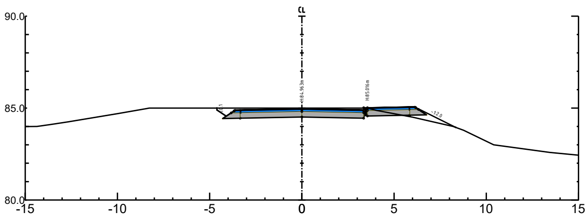
o_V1 Pel nr 80 - Skala 1:500
