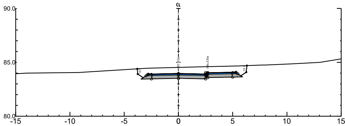
o_V1 Pel nr 190 - Skala 1:500
