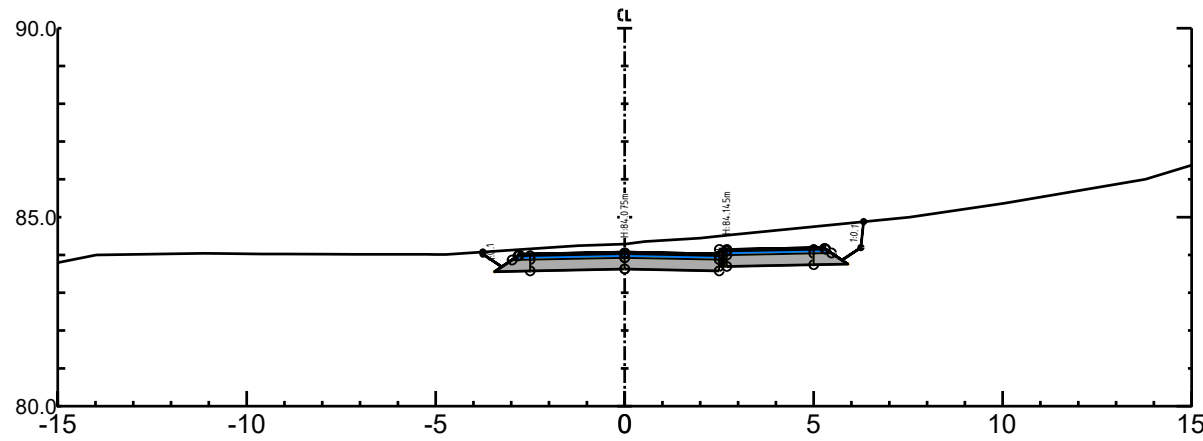
o_V1 Pel nr 200 - Skala 1:500
