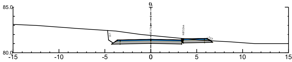
o_V1 Pel nr 30 - Skala 1:500
