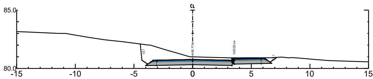
o_V1 Pel nr 20 - Skala 1:500
