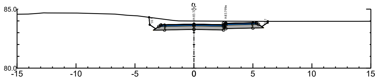
o_V1 Pel nr 160 - Skala 1:500
