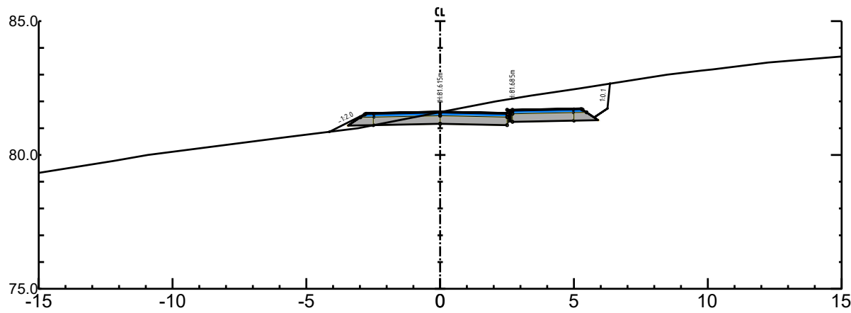
o_V1 Pel nr 420 - Skala 1:500
