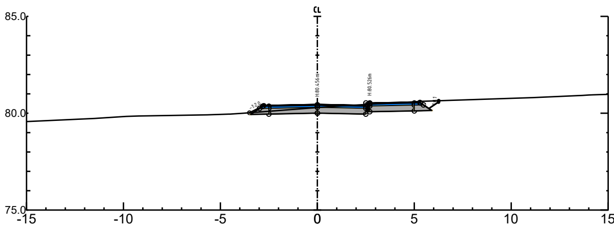
o_V1 Pel nr 330 - Skala 1:500
