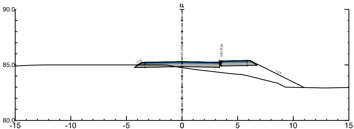
o_V1 Pel nr 90 - Skala 1:500
